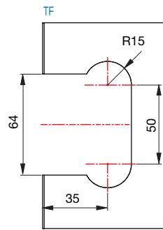
Glasbearbeitung/ glass processing
