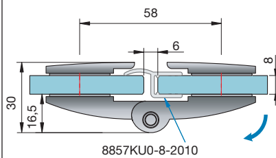
8122ZN mit Dichtprofil 8857KU0-8-2010 8122ZN with sealing profile 8857KU0-8-2010
