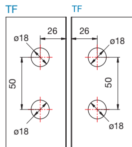
Glasbohrung glass bore
