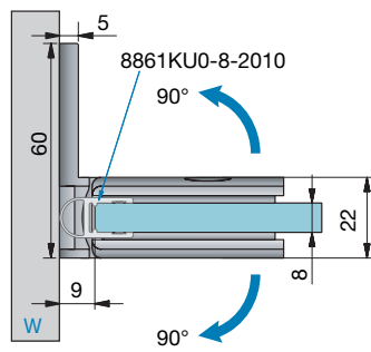
8406MS mit Dichtprofil 8861KU0-8-2010 8406MS with sealing profile 8861KU0-8-2010
